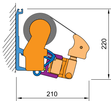
Montáž do stěny
