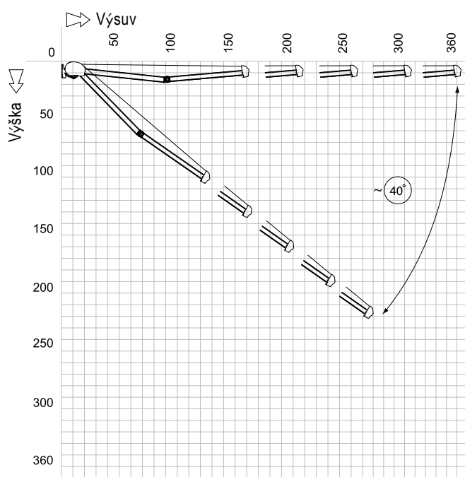
Rozsah regulace sklonu markýz
