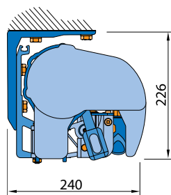
Montáž do stropu
