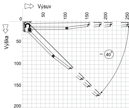
Rozsah regulace sklonu markýz
