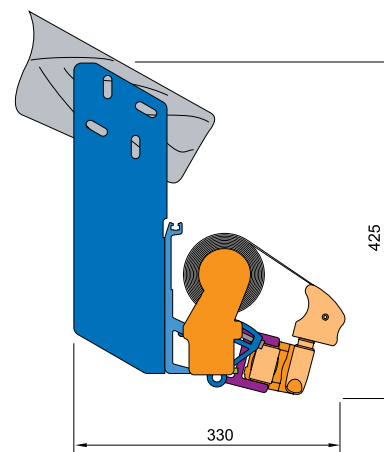
Montáž do krovu
