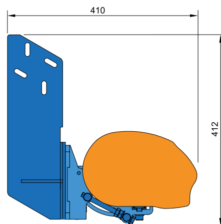
Montáž do krovu
