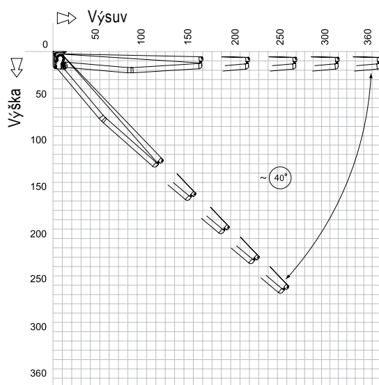
Rozsah regulace sklonu markýz
