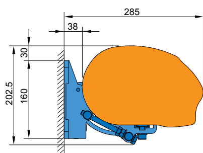
Montáž do stěny
